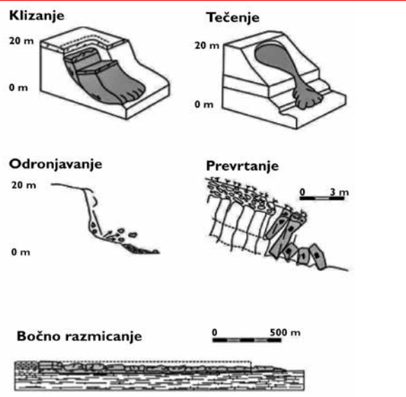
Slika 2. Tipovi klizišta
